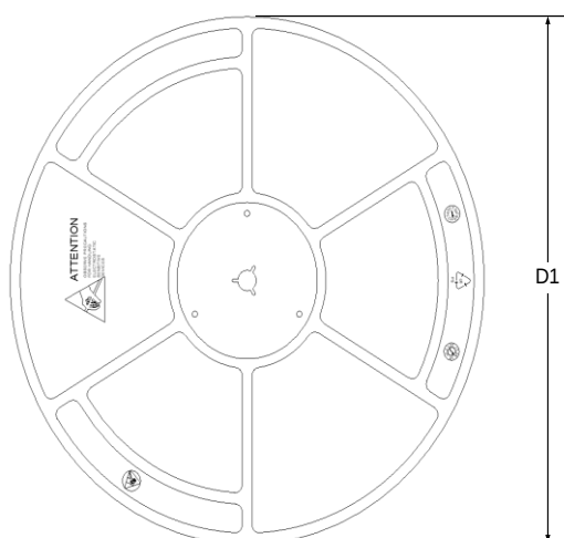
REEL DIMENSIONS
